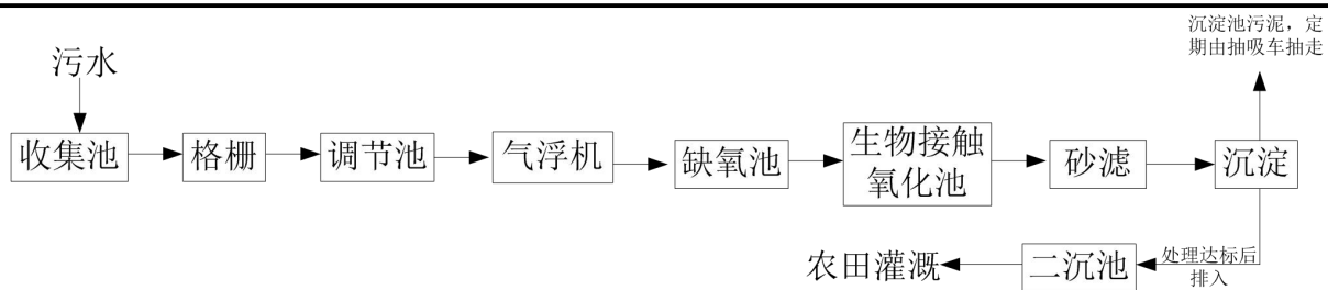
图4 污水处理站工艺流程图
