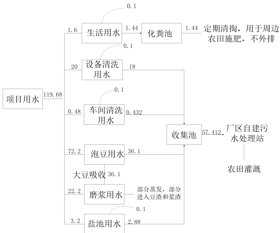
图1 项目营运期水平衡图 单位: t/d
