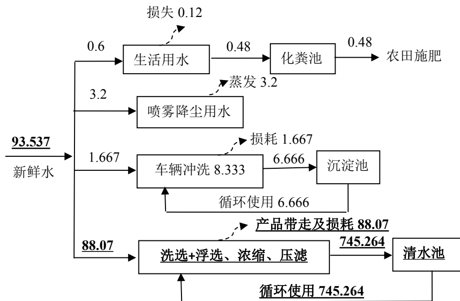
图 1 项目运营期水平衡图 单位：t/d
