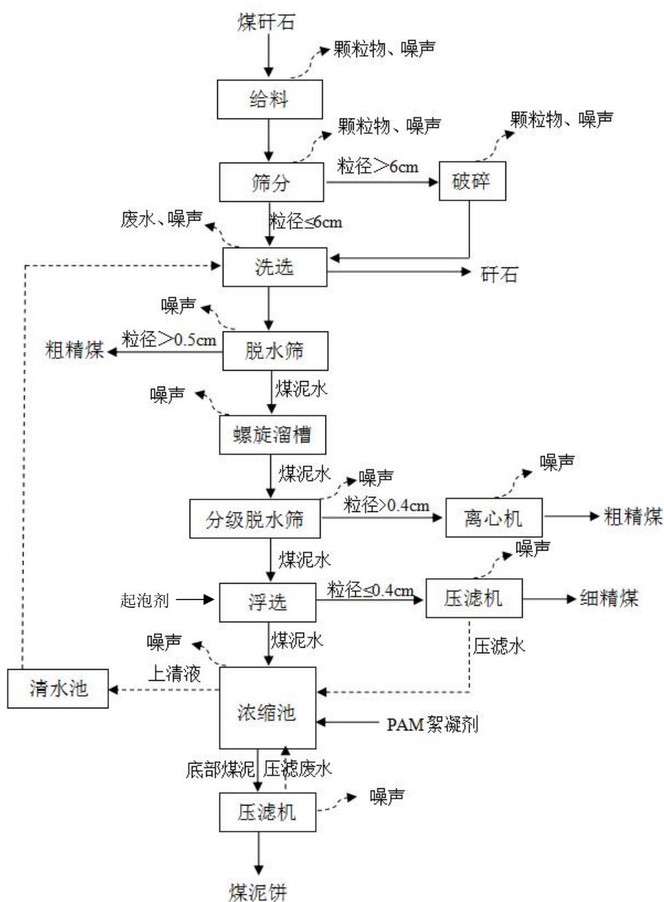
图3 营运期工艺流程及产污环节示意图
