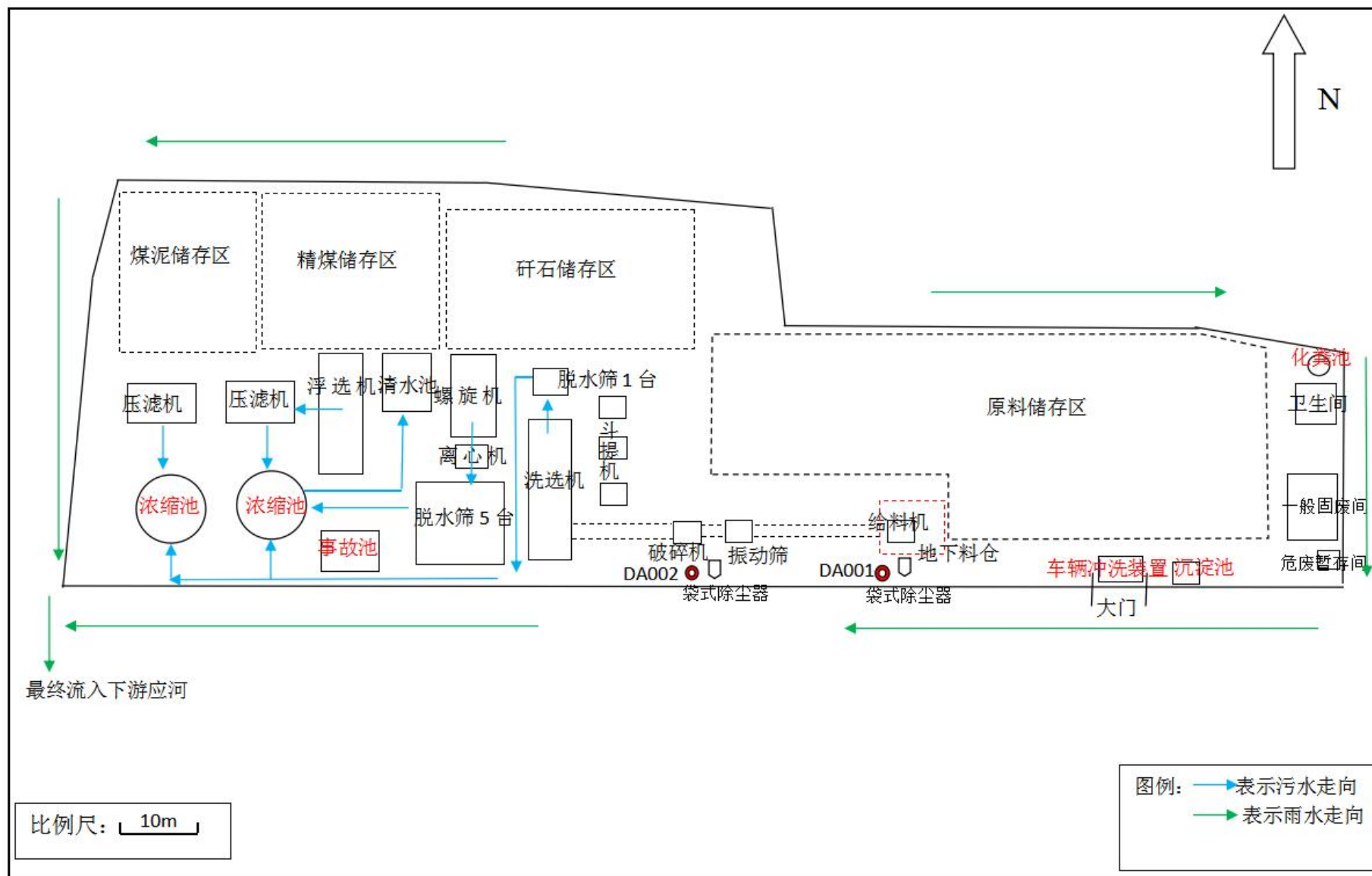
附图六 项目雨污分流及走向图
